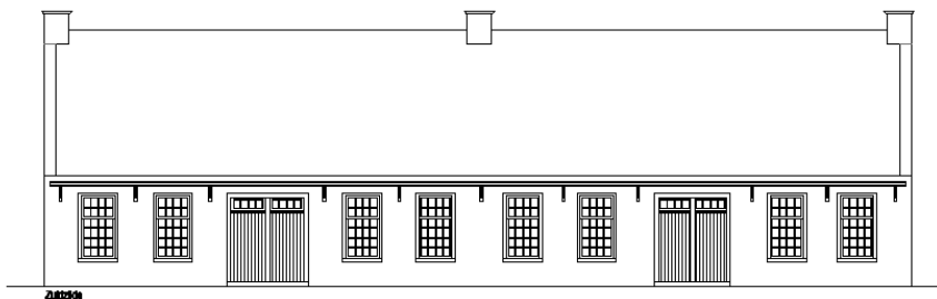
Voorgevel van het gasthuis, getekend naar het bestek door Jacob van Wolde, naar het oude bestek.
